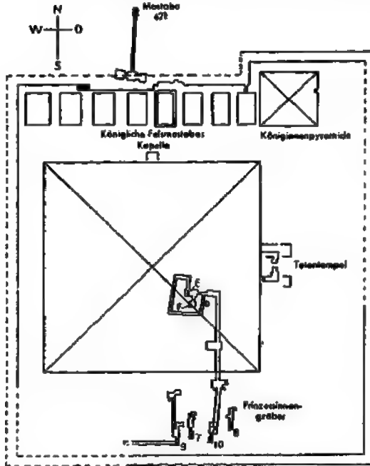
مسقط أفقى للمجموعة الهرمية لسنوسرت الثاني «حوالى ١٨٩٠ ق. م» في اللاهون
